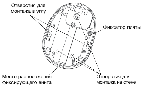
Рисунок 2 – Основание извещателя
